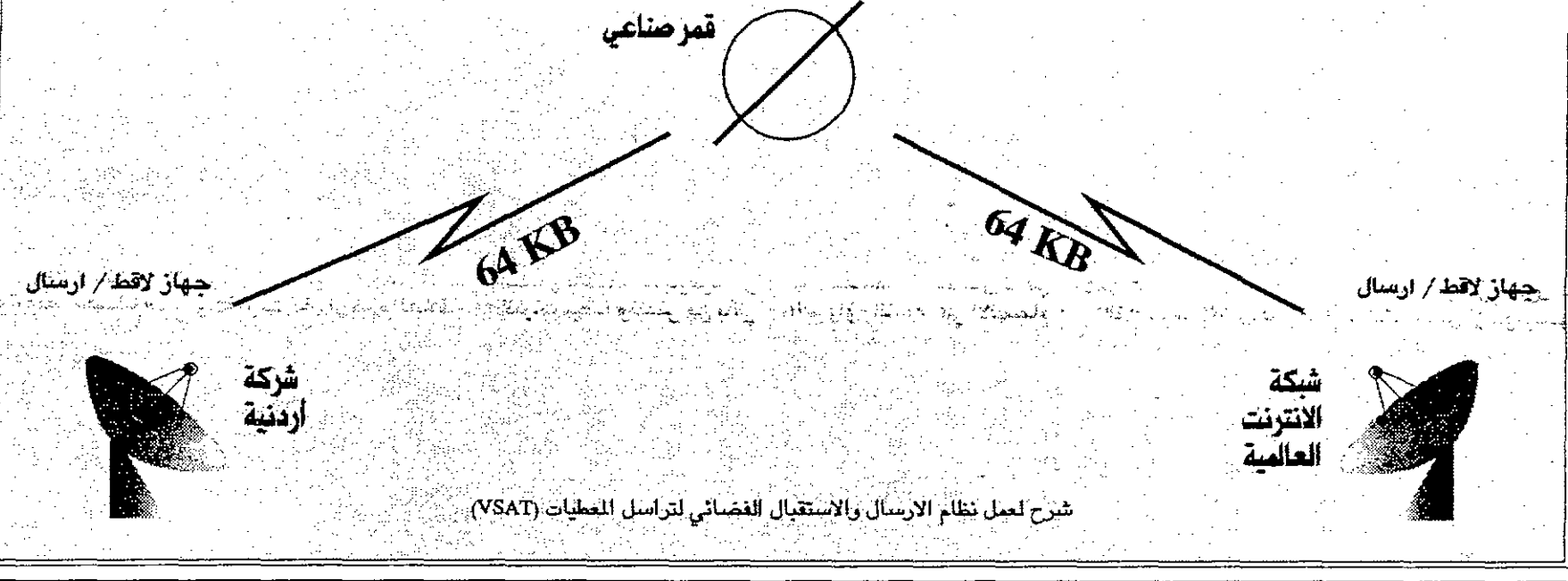
شرح لعمل نظام الارسال والاستقبال الفضائي لتراسل المعطيات (VSAT)
